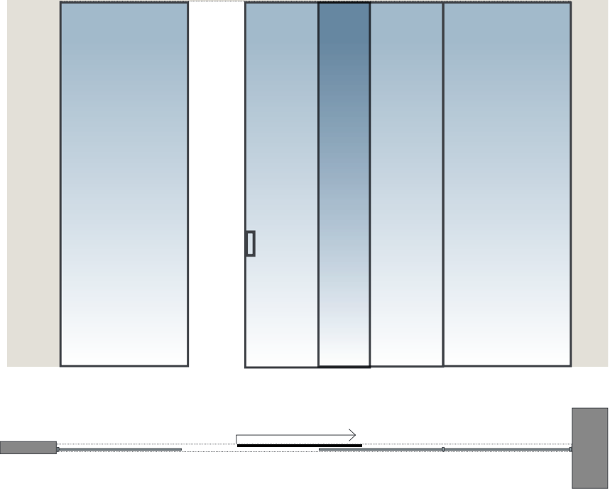
Porta scorrevole su parete composta a tutt'altezza e binario a scomparsa
